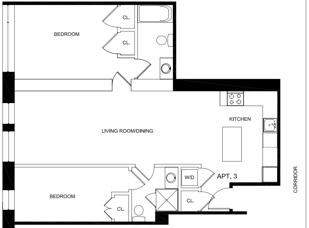
1 APARTMENT #3 A-2 SCALE: 1/8" = 1'-0"
